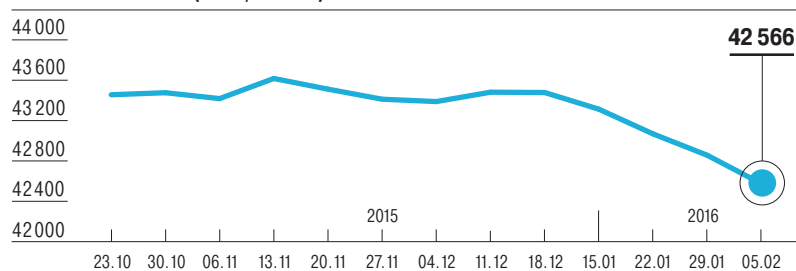
ЦЕНЫ НА АВИАЦИОННЫЙ КЕРОСИН В НЕКОТОРЫХ АЭРОПОРТАХ РФ НА 15 ЯНВАРЯ 2016 ГОДА (РУБ./ТОННА) ИСТОЧНИК: РОСАВИАЦИЯ.
