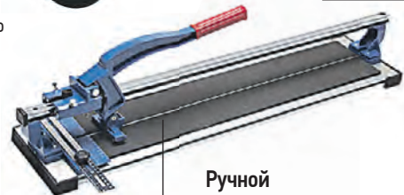
Ручной плиткорез Служит для фигурных резов в плитке и стекле до 8 мм толщиной. Это простой и удобный инструмент, чтобы выполнять нестандартные углубления, например, под выступающий плинтус или вентиляционную трубу и прочее.
